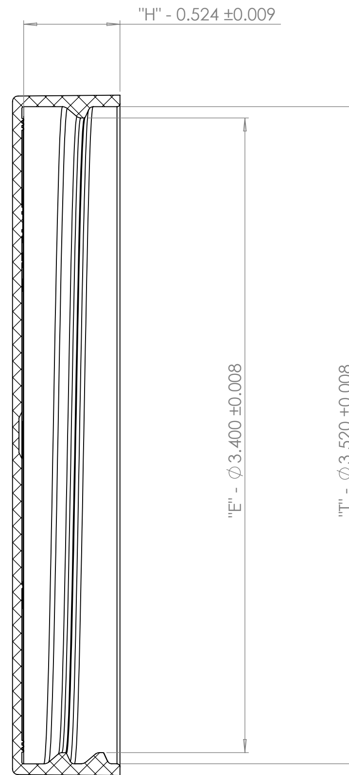
SECTION A-A
